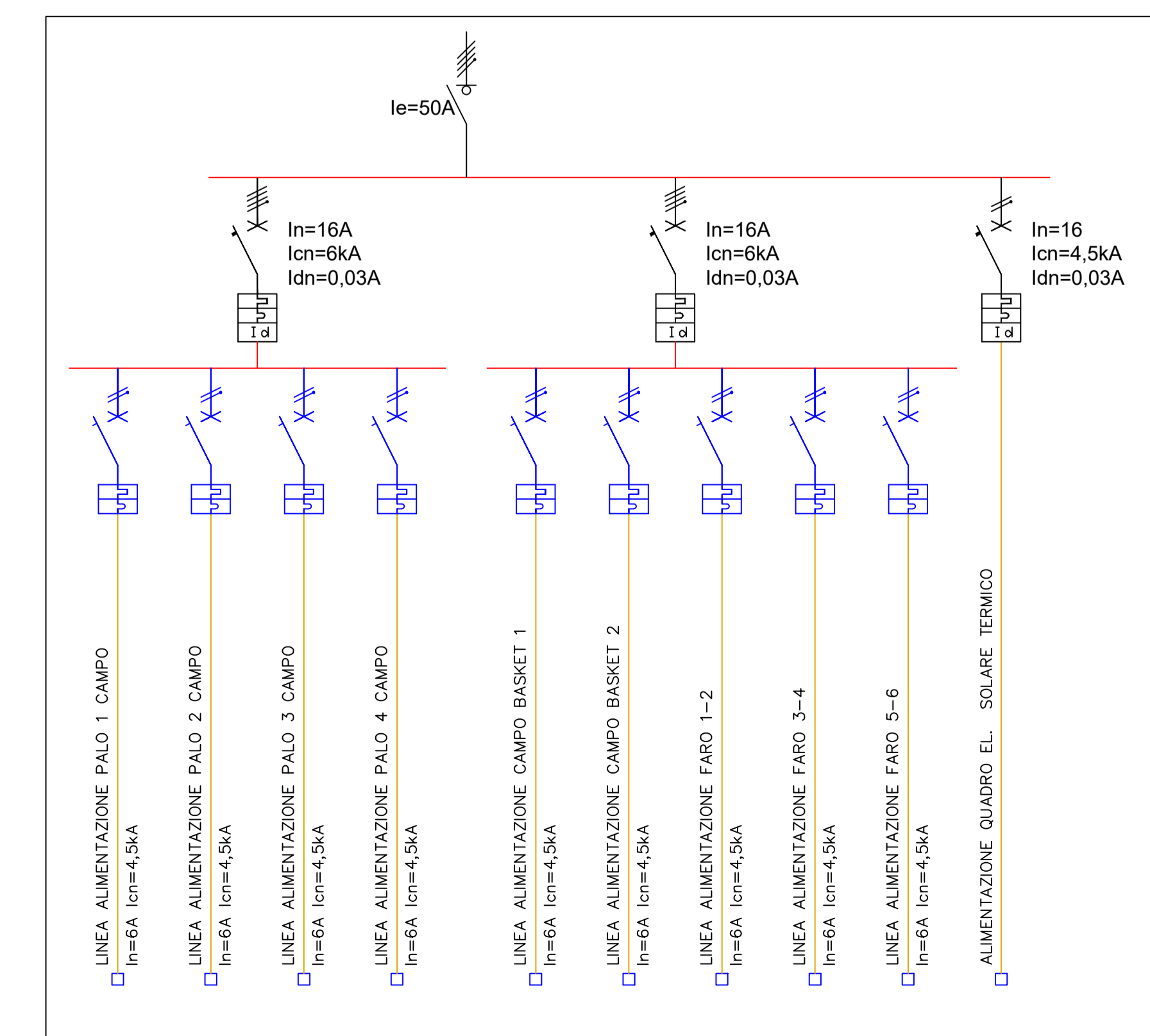
QUADRO ELETTRICO ILLUMINAZIONE CAMPI DA GIOCO
