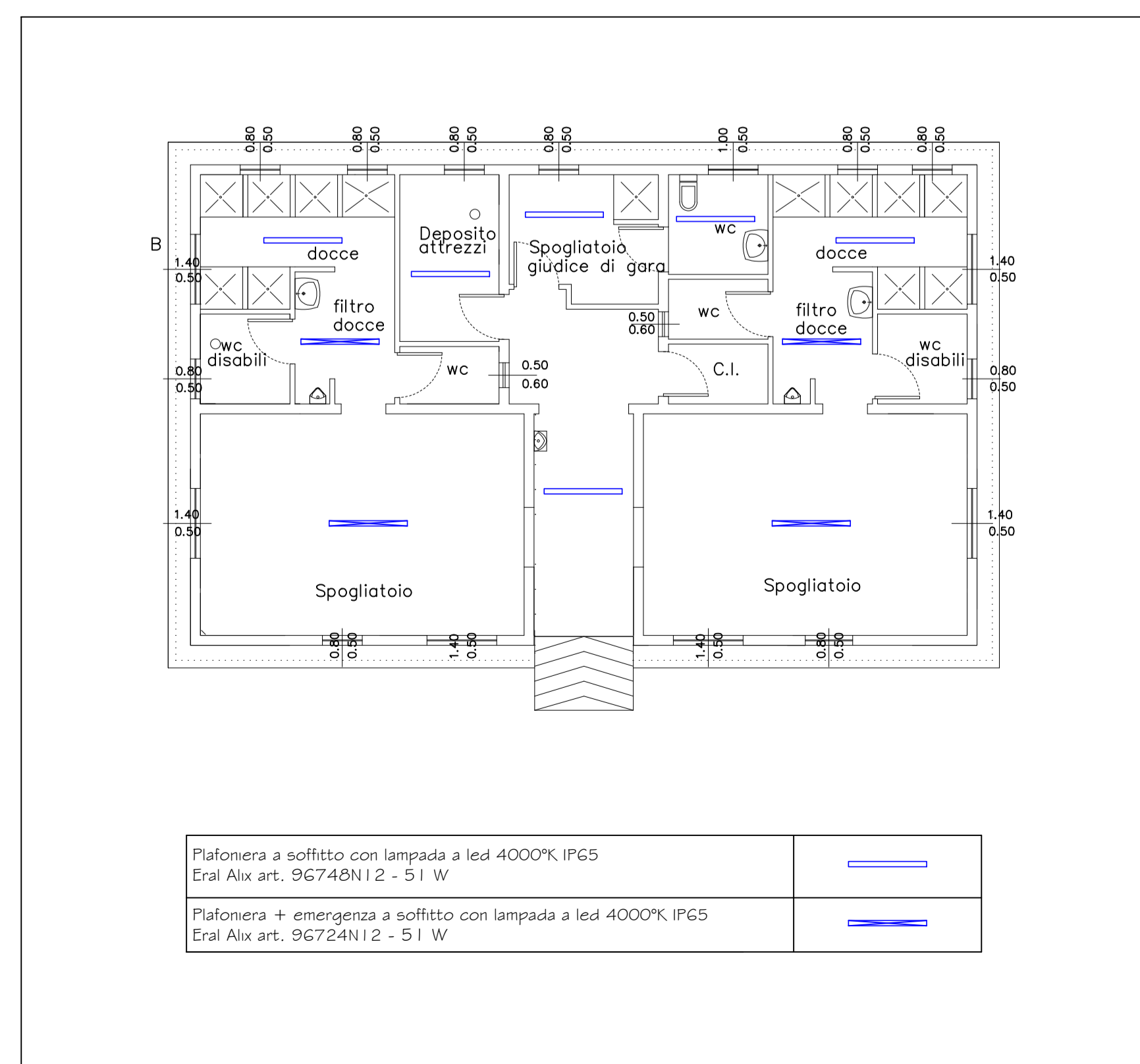
DETTAGLIO A RELAMPING - PIANTA SPOGLIATOI 1:100
